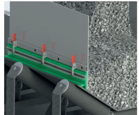
Bavette d'étanchéité
